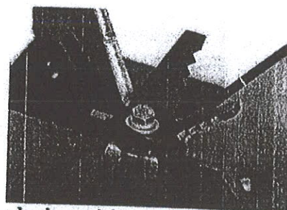
PIRANHA kések - dupla aprítás - tömörebb apríték
